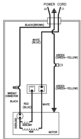
以下型號的配線圖 "N222, V222, BL222, E222"
