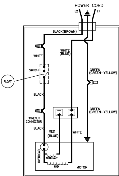
以下型號的配線圖 "WM222, WU222, WB222, WD222"
